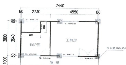
2K*4K*3P(平面图)
