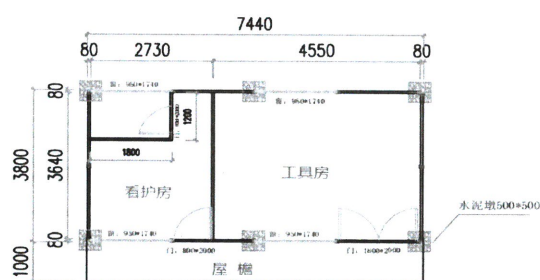
2K*4K*3P(平面图)
