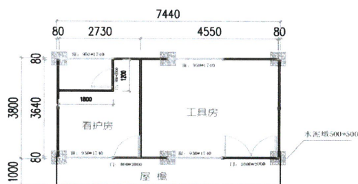
2K*4K*3P(平面图)
