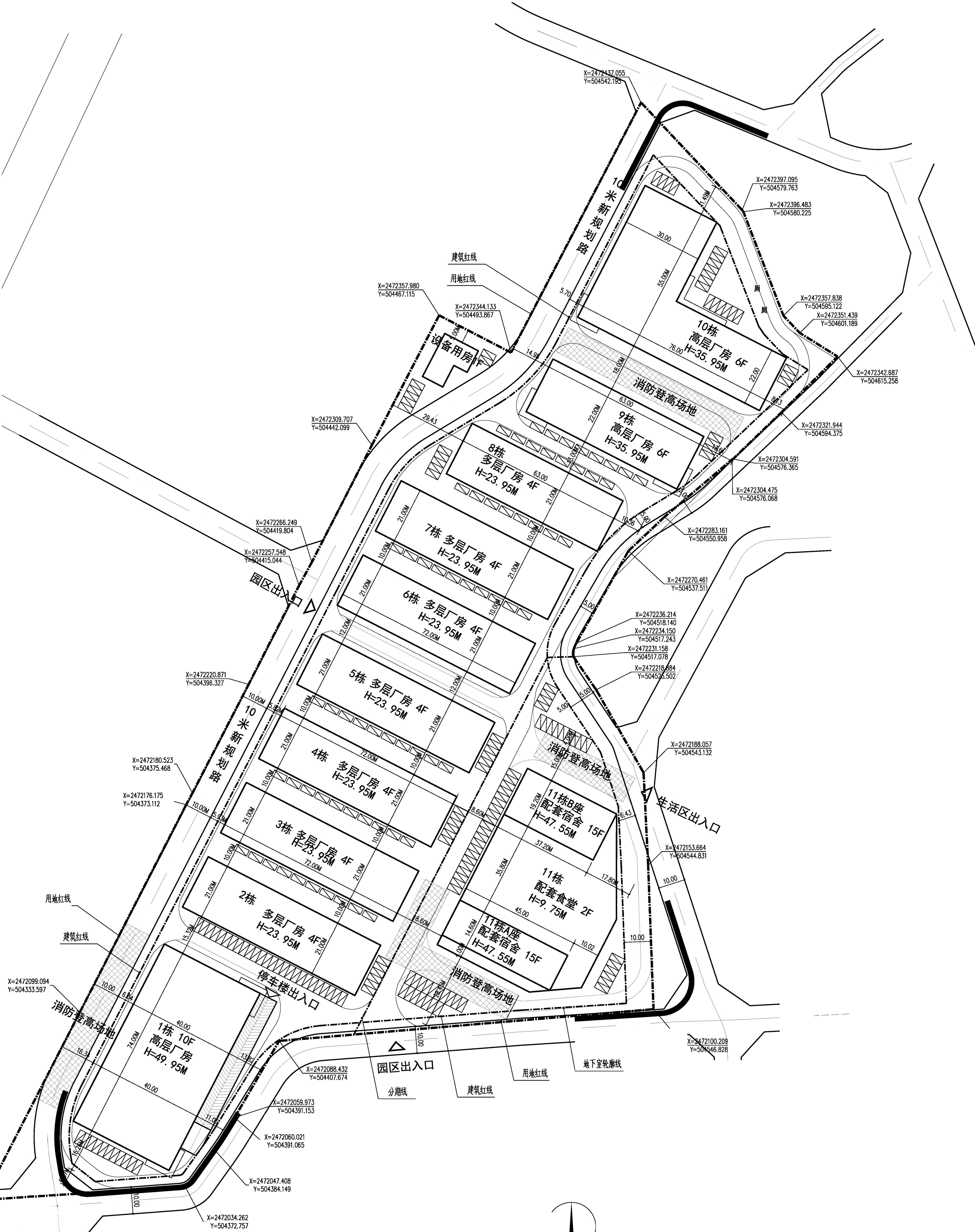
总平面图 1:1000
