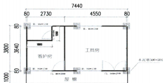
2K*4K*3P(平面图)
