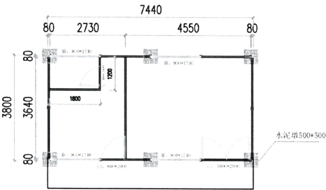
2K*4K*3P(平面图)
