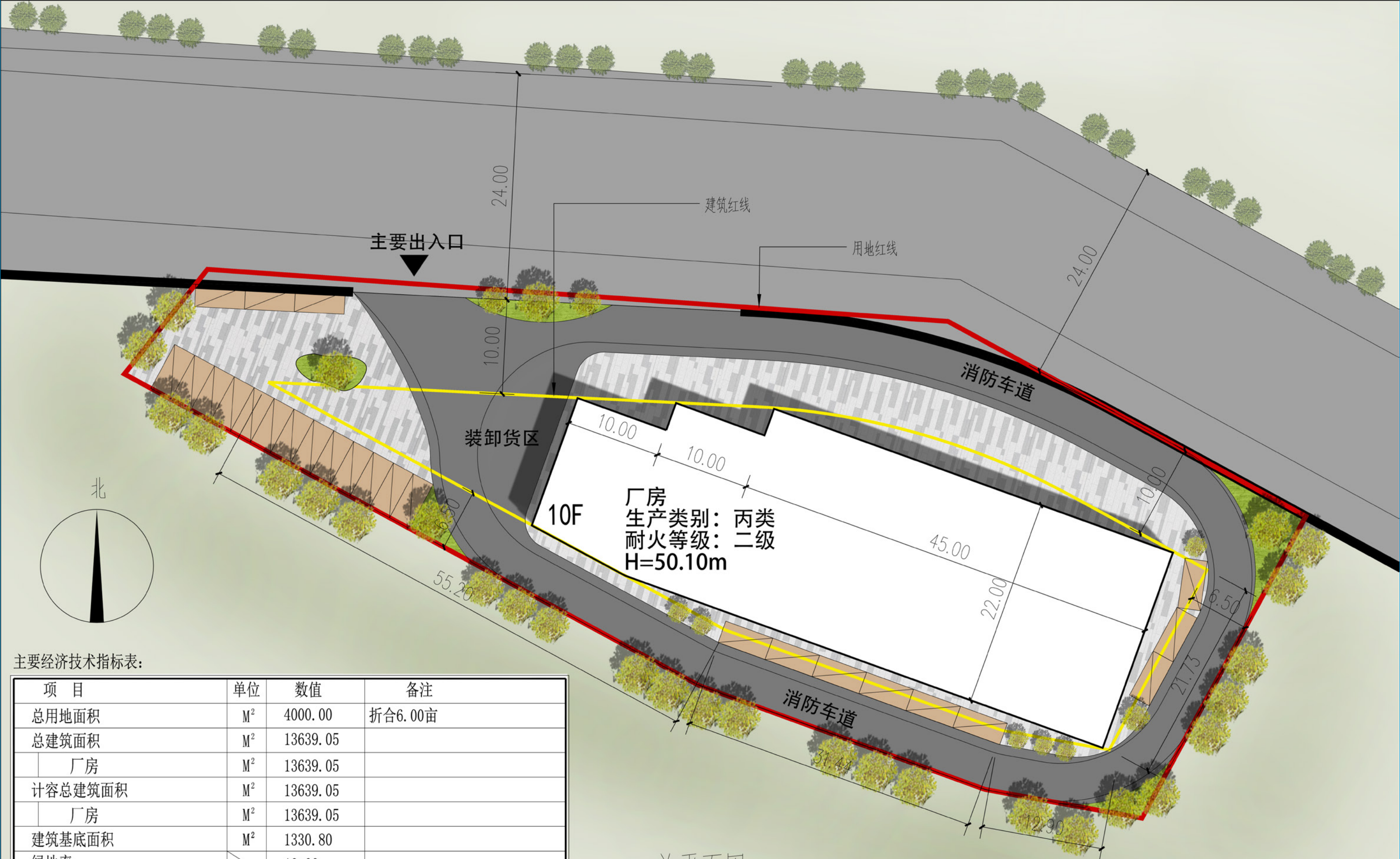
总平面图 1:500
