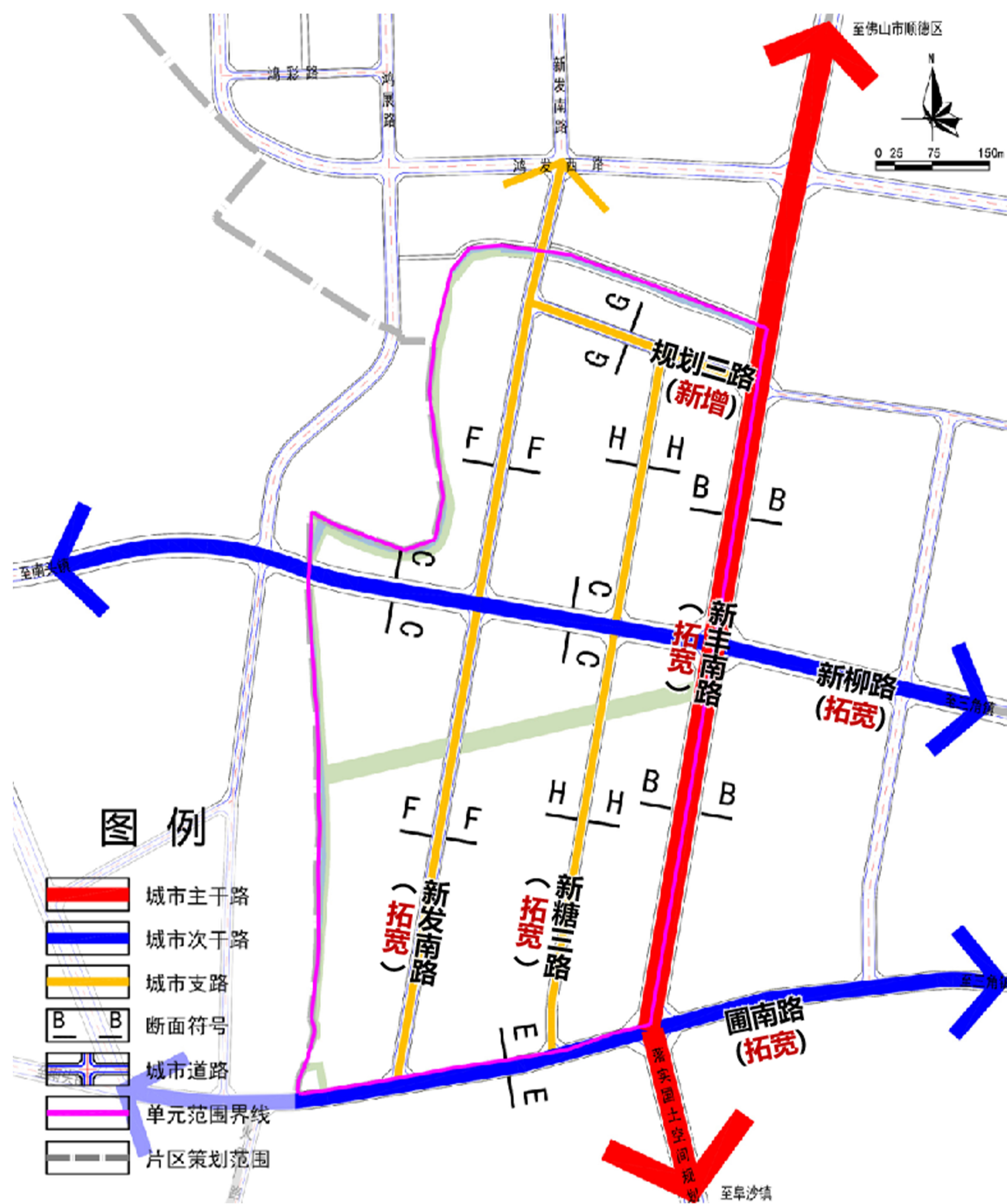
道路交通系统规划图
