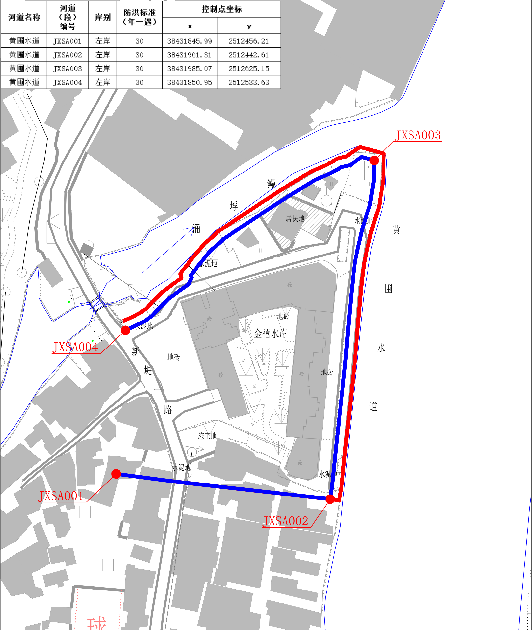
黄圃水道金禧水岸河段管理范围线平面布置图
