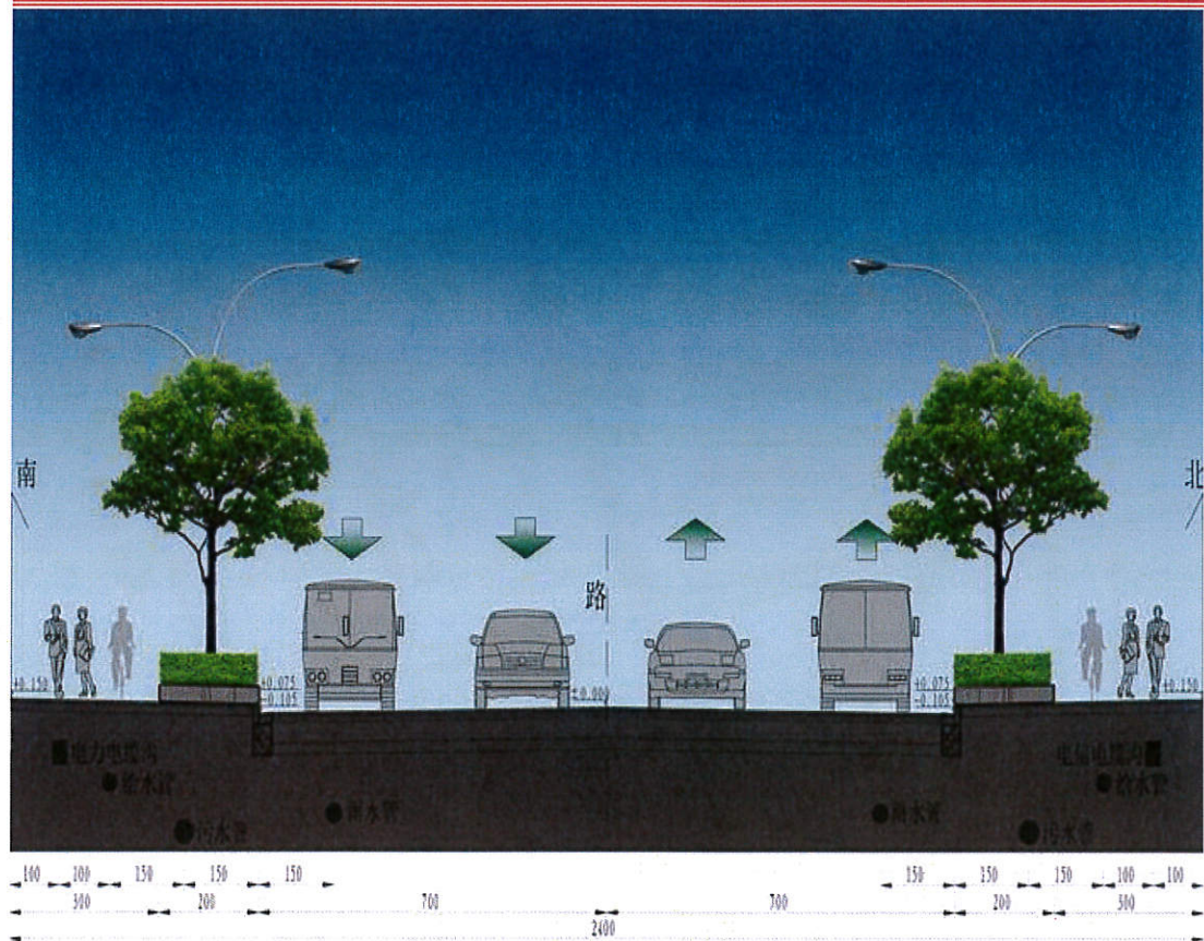
24米单幅路标准横断面图 1: 100
