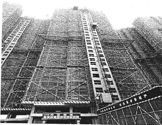
15 栋（屋面花架柱钢筋绑扎施工中）
