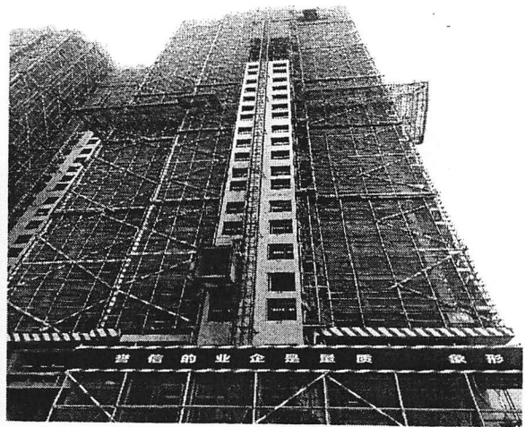
8 栋（三十二层柱钢筋绑扎施工中）
