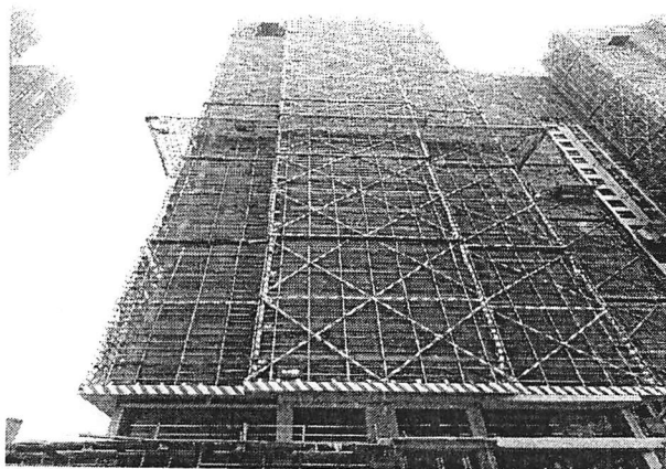
5 栋主楼 (三十二层柱钢筋绑扎施工中)
