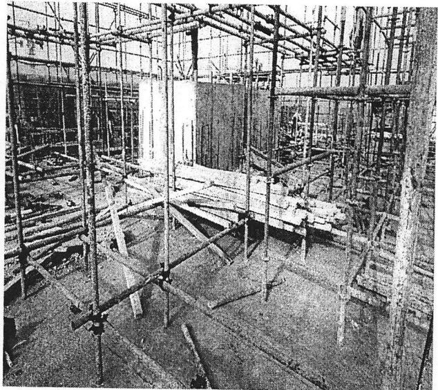
12 栋（屋面砼浇筑完成）
