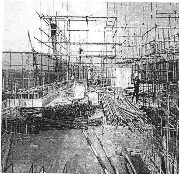
11 栋（屋面砼浇筑完成）
